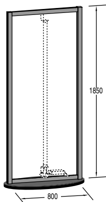
рама световой колонны
